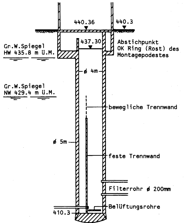
Pumpschacht mit horizontalen Fassungssträngen
